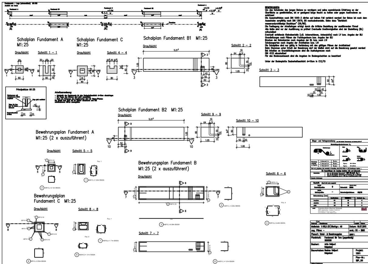
Schal- & Bewehrungsplan
