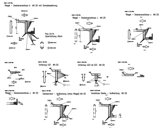
Bewehrungsplan Decke EG (Details)
