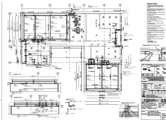
Bewehrungsplan Decke EG
